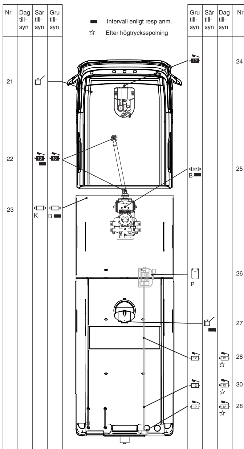
Bild 2. Påbyggnad
