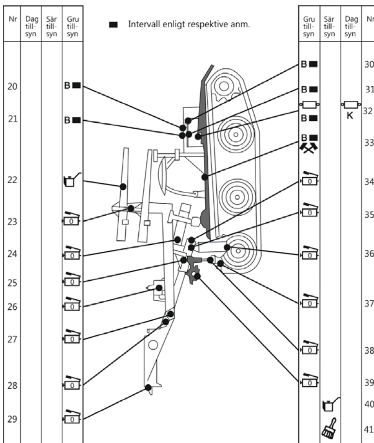
Bild 2. Laddbandvagn 912B
