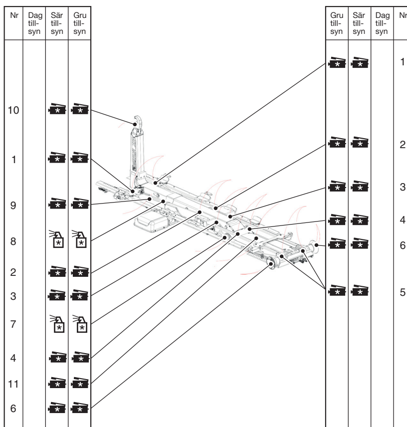
Bild 2. Rullflaksväxlare
